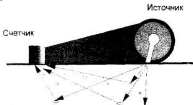
Рис. 5. Схема поверхностного просвечивания (рассеяния)
