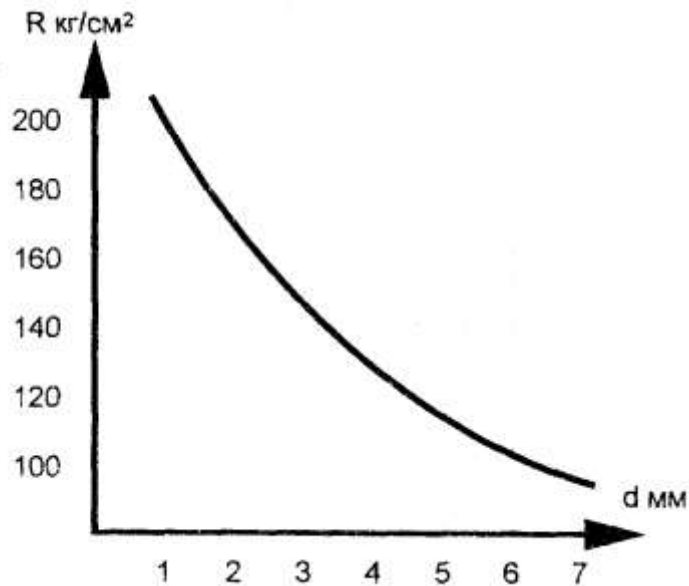
Рис.1 Тарировочная зависимость размера отпечатка от прочности бетона
